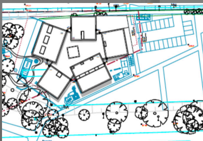
Grundriss Gelände
